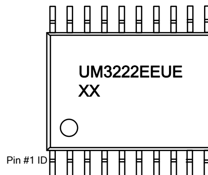
XX: Week Code UM3222EEUE TSSOP20
