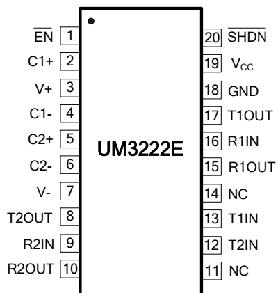
TSSOP20
